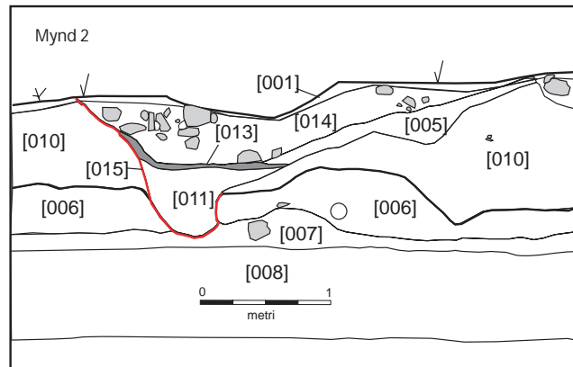
Mynd 2 Sniðteikning af niðurgrefti [015].
